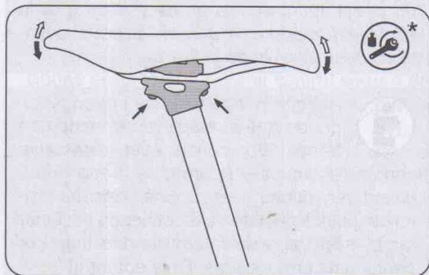
Tija con mecanismo de sujeción integrado con dos tornillos
