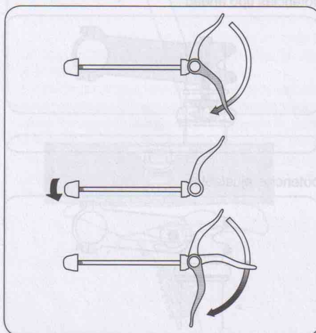
Apretar la tuerca de reglaje
